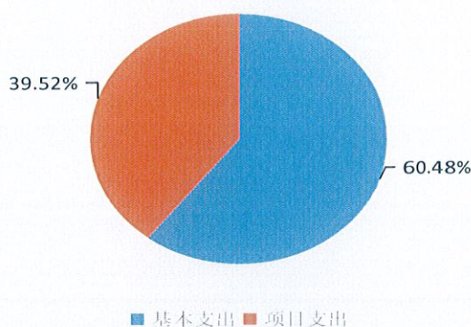
图3: 支出决算(单位:万元)
